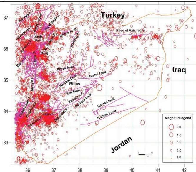
شكل 2. النشاط الزلزالي في سورية وجوارها كما وثقته الشبكة الوطنية للرصد الزلزالي من 1995 وحتى 2012 (Abdul-Wahed and Asfahani, 2018).
