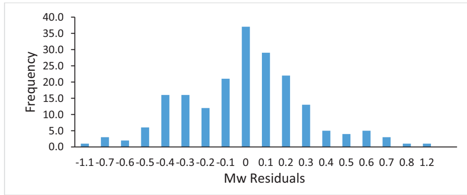
شكل 4. هيستوغرام الفروقات بين قدر الطاقة ( M_w ) المحسوب من العلاقة التجريبية بين قدر الطاقة ( M_w ) والملاحظ في قاعدة المعطيات قدر الهزات المحلية ( M_L ).
