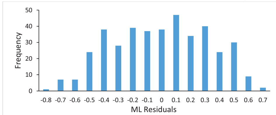
شكل 9. نتائج العلاقة التجريبية بين قدر الزلازل المحلية ( M_L ) وقدر نهاية التسجيل ( M_C ).
