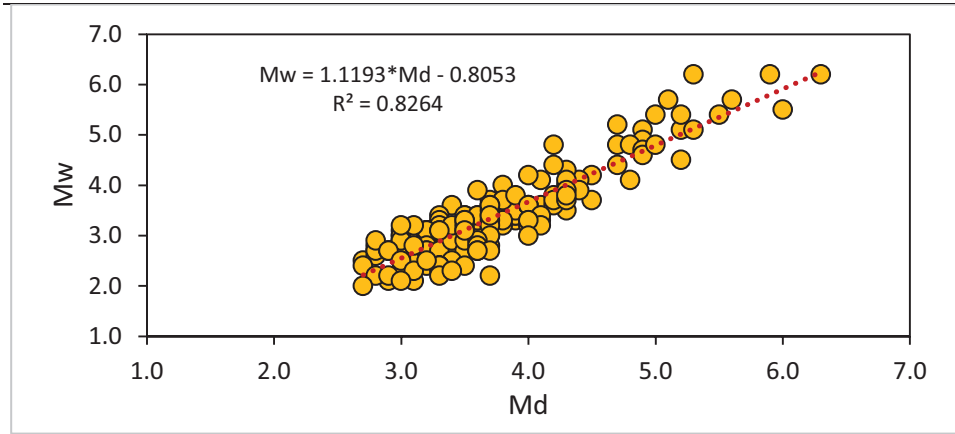
شكل 5. نتائج العلاقة التجريبية بين قدر الطاقة ( M_w ) وقدر المدة ( M_d ).
