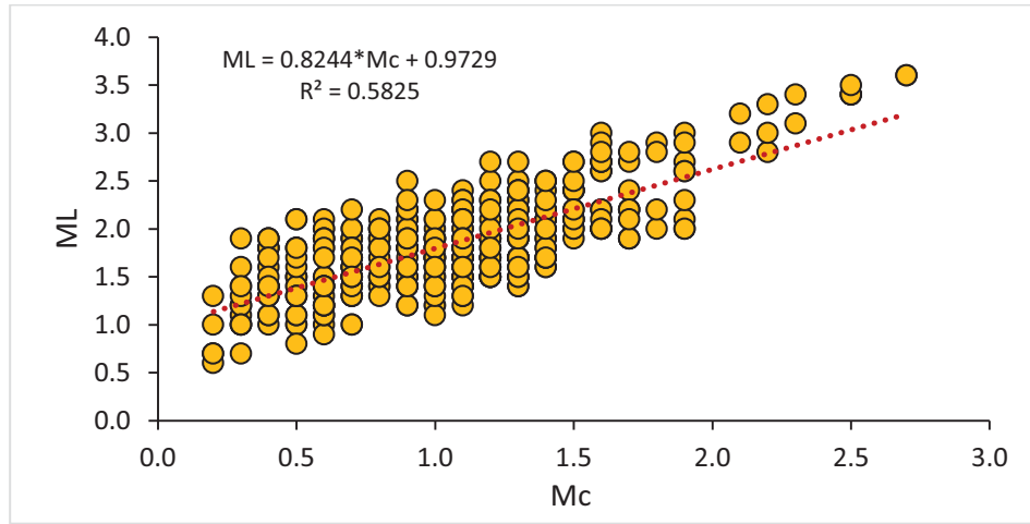
شكل 9. نتائج العلاقة التجريبية بين قدر الزلازل المحلية ( M_L ) وقدر نهاية التسجيل ( M_C ).
