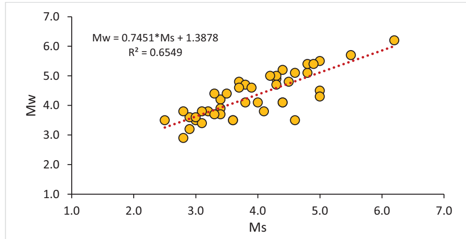
شكل 7. نتائج العلاقة التجريبية بين قدر الطاقة ( M_w ) وقدر الأمواج السطحية ( M_s ).
