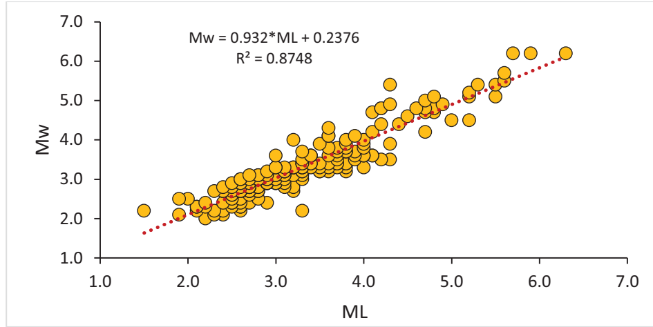
شكل 3. نتائج العلاقة التجريبية بين قدر الطاقة ( M_w ) وقدر الهزات المحلية ( M_L ).
