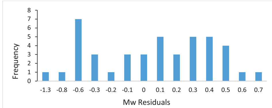
شكل 8. هيستوغرام الفروقات بين قدر الطاقة ( M_W ) المحسوب من العلاقة التجريبية بين قدر الطاقة ( M_W ) الملاحظ في قاعدة معطيات قدر الأمواج السطحية ( M_S ).
